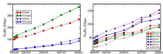
各グループのトラフィック推移-顧客側(左)外部ISP側(右)
